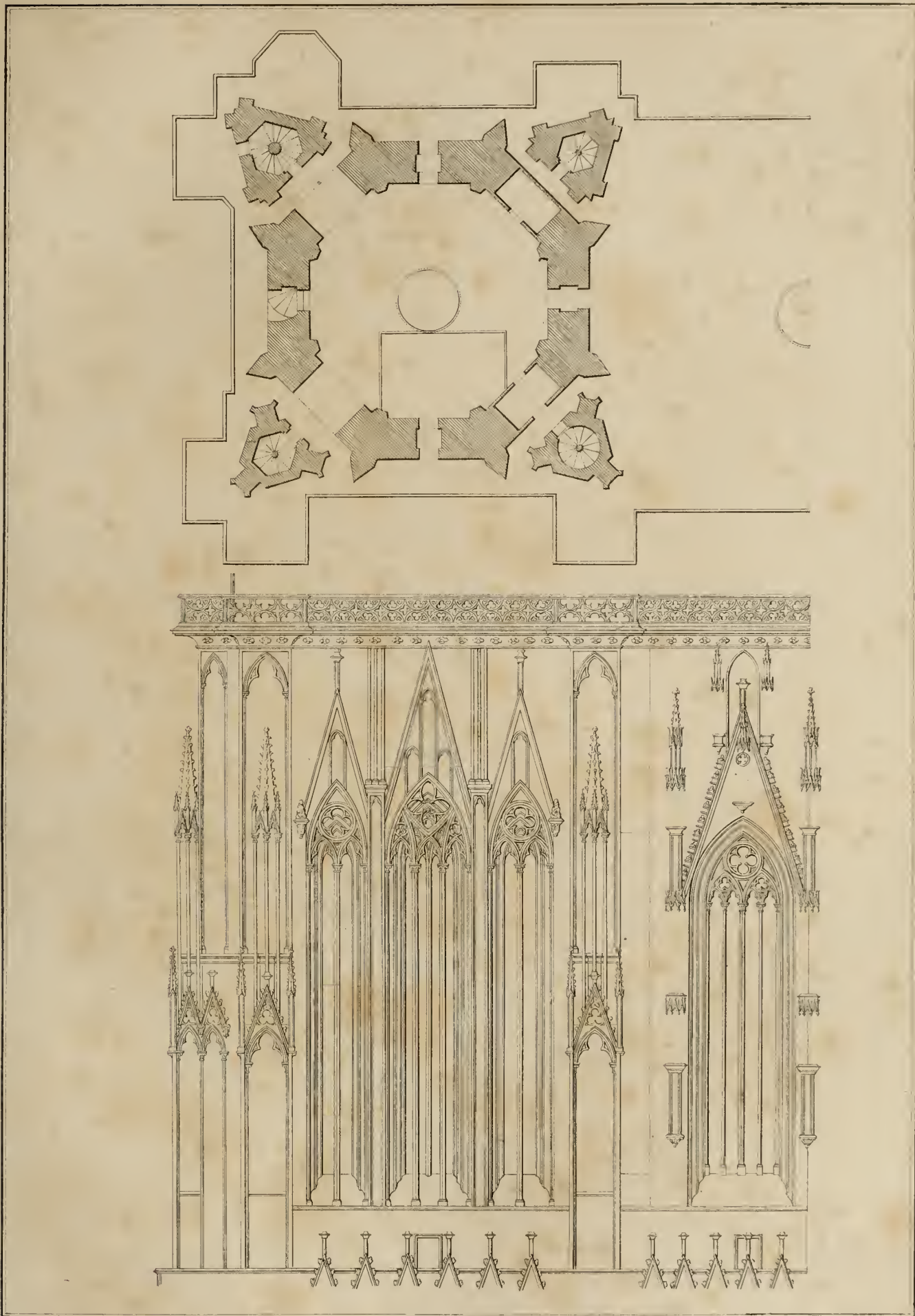
Elevation géométrale (Partie supérieure de la façade et plan de la tour.)
